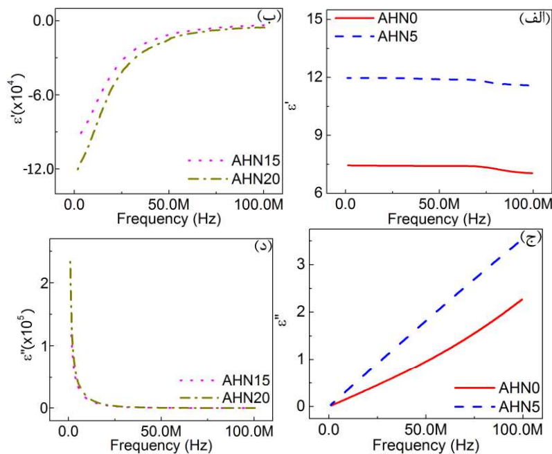
شکل ۳ تغییرات گذردی (الف) و (ب) حقیقی، (ج) و (د) موهومی بر حسب بسامد مربوط به نمونه‌های با مقدار نقره ۰، ۵، ۱۵ و ۲۰ درصد.
