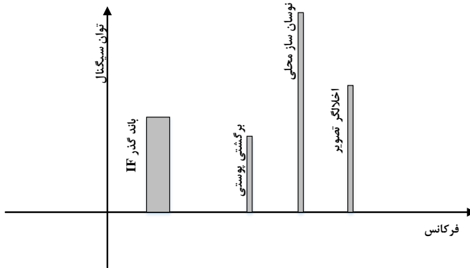
شکل (۱۱) نمودار طیف فرکانسی در گیرنده سوپرهتروداین
