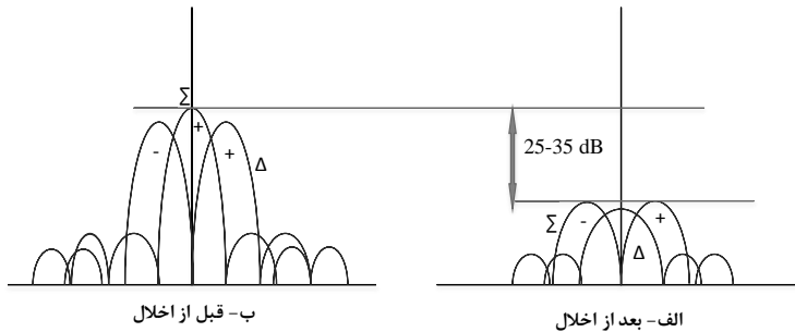
شکل (۱۴) الگوهای جمع و تفاضل در رادار مونوپالس قبل و بعد از اخلاص قطبش متقاطع
