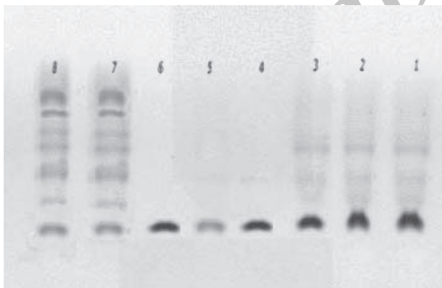
شکل ۲-۱، ۳ و ۴ - نمونه های تریپسین استحصال شده با روش Wilimowska. ۶۴ - نمونه های تریپسین تخلیص شده با روش این مطالعه. ۵ - نمونه تریپسین کمپانی فلوکا. ۷ و ۸ - نمونه های تریپسین استحصال شده از روش Kuintz
