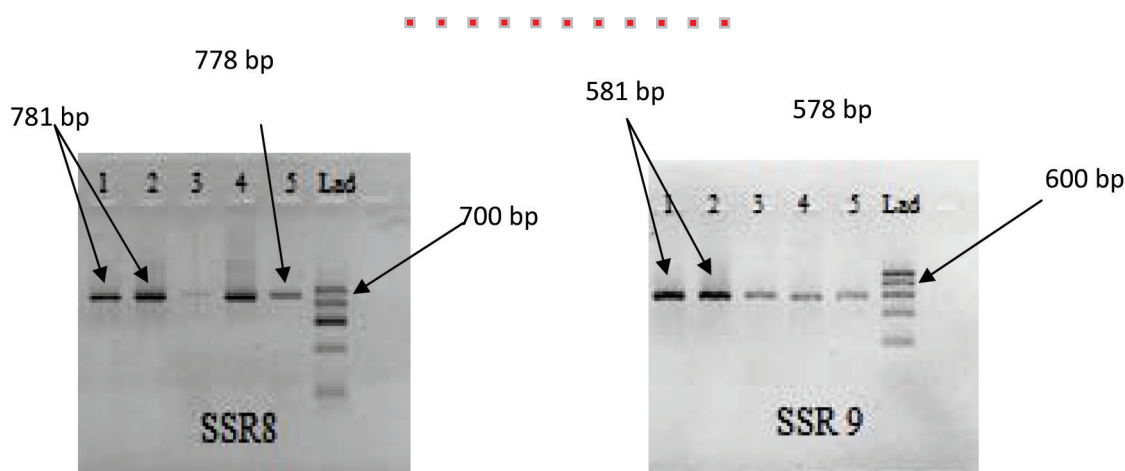
تصویر ۱) الکتروفورز محصولات PCR مربوط به لوکوس های SSR9 و SSR8 بر روی ژل آگاروز ۲.۱. ستون شماره Razi 01911 1، ستون شماره 2Razi 01450، ستون شماره ۳ Razi 01231 مربوط به جدایه های ایرانی و ستون شماره ۴ معرف سویه V و PAM III می باشند. DNA size marker بکار رفته دارای ۵ باند الکتروفورز به فواصل 200 bp در محدوده 100 الی 900 (SSR8) یا 200 الی 1000 (SSR9) می باشد.
