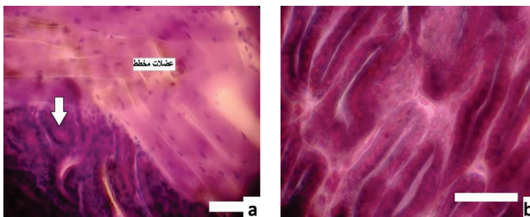
شکل ۵- (a) میکروگراف نوری غده کوپر گروه نهان بیضه. کاهش جزئی آلوئولهای ترشچی (فلش سفید رنگ) مشاهده می‌گردد (رنگ آمیزی Oil Red O، درشت‌نمایی ۴۰ برابر)، (b) میکروگراف نوری غده کوپر گروه نهان بیضه. عدم مشاهده واکنش مثبت به چربی (رنگ آمیزی سودان بلک، درشت‌نمایی ۴۰ برابر).
