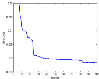
شکل ۵ روند همگرایی در بهینه‌سازی ازدحام ذرات (PSO)
