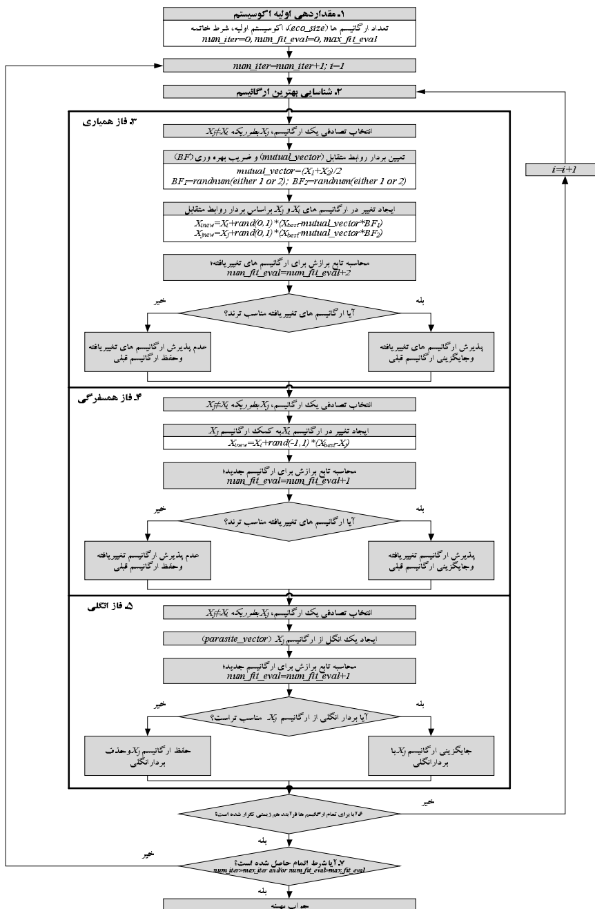
شکل ۴ الگوریتم جستجوی ارگانیسم‌های همزیست
