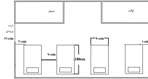
شکل ۵: نمای شماتیک اتاقها قبل از مداخله
