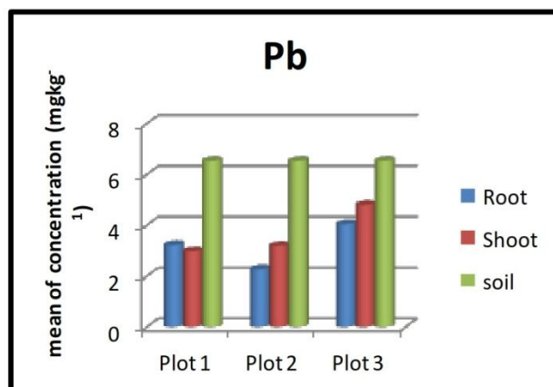
نمودار ۳. میانگین غلظت فلزات سرب و نیکل در ریشه، اندام هوایی و خاک هر پلات به طور جداگانه
