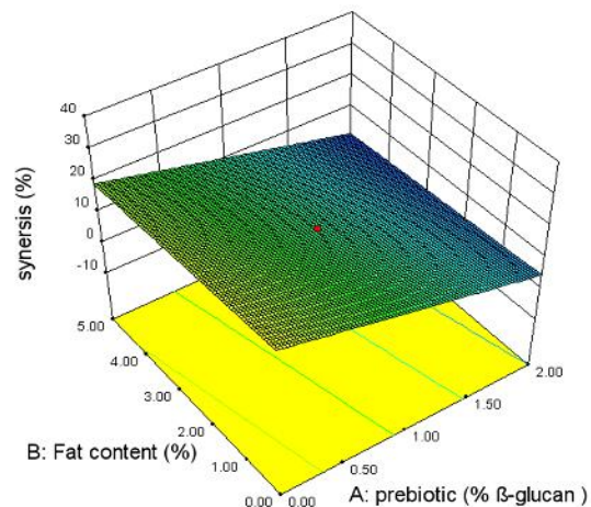
شکل ۲. نمودار سه‌بعدی برای بررسی میزان آب‌اندازی بر اثر تغییر در درصد β-گلوکان و درصد چربی
