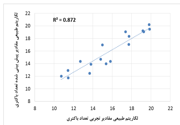
شکل ۸. مقایسه مقادیر تجربی تعداد باکتری و مقادیر پیش‌بینی شده توسط شبکه عصبی مصنوعی
