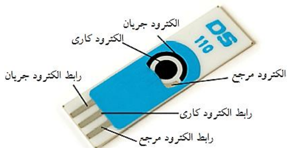
شکل ۱. الکتروود نمونه صفحه چاپی (الکتروود پایه کربنی)
