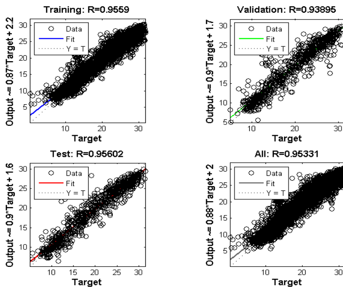
شکل ۶- خروجی شبکه ANN6-2 برای داده‌ها (منبع: خروجی نرم افزار متلب)
