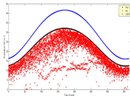
شکل ۳- داده‌های تشعشع پس از غربال‌گری (منبع: داده‌های ایستگاه هواشناسی مشهد)
