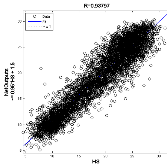
شکل ۱۰- خروجی ANN6-2 در مقایسه با HS (منبع: خروجی نرم افزار متلب)
