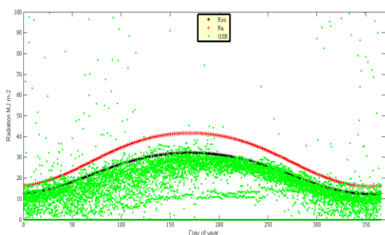
شکل ۲- داده‌های اولیه تشعشع قبل از غربال‌گری (منبع: داده‌های ایستگاه هواشناسی مشهد)
