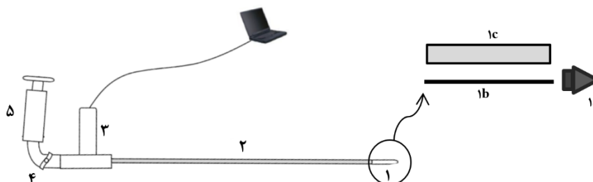
شکل ۱- حسگر بولینگ و اجزاء تشکیل دهنده: ۱- هد حسگر، ۲- لوله PVC، ۳- حسگر دیجیتال فشار، ۴- شیر کنترل حجم آب و ۵- سرنگ پرکن. قسمت بزرگنمایی شده اجزاء هد حسگر را نشان می‌دهد: ۱a مخروط آلومینیومی، ۱b مفتول آهنی و ۱c شلنگ لاستیکی.
