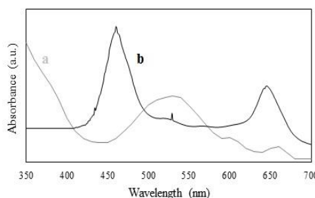
شکل ۳. طیف جذبی UV-Vis محلول رنگدانه استخراجی از پوست سبز گردو و محلول رنگدانه جذب شده بر روی نانوذرات دی اکسید تیتانیوم (a)، (b).
