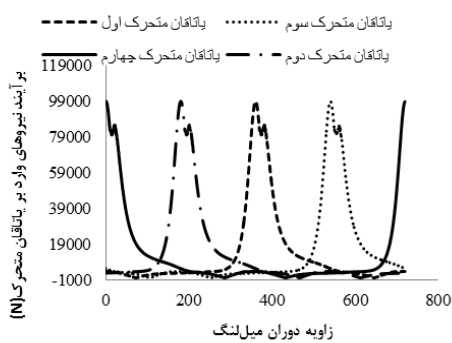
شکل ۲. نیروهای مؤثر بر پیستون و یاتاقان متحرک سیلندر یک در سرعت دورانی ۱۳۰۰rpm (الف) و ۲۲۰۰ (ب)
