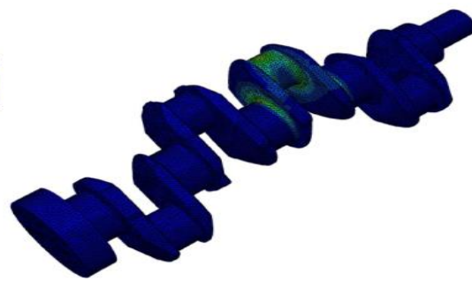
شکل ۸. توزیع تنش وان میسز در سرعت دورانی ۲۲۰۰ دور بر دقیقه ۱ درجه بعد از احتراق سیلندر ۱، ۲، ۳ و ۴ برحسب مگا پاسکال
