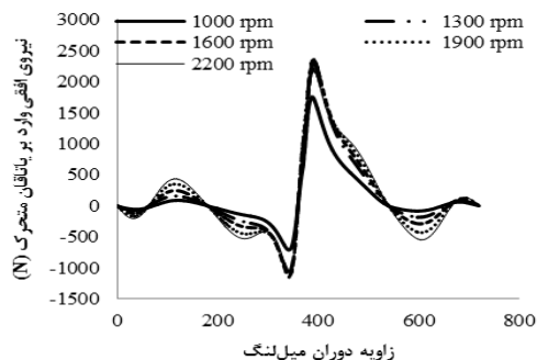
شکل ۱. نمودار تغییرات نیروی افقی وارد بر یاتاقان متحرک
