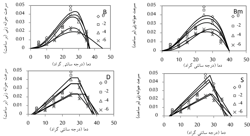
شکل ۲- رابطه سرعت جواهر زنی با دما در پتانسیل‌های مختلف آب با استفاده از مدل‌های بتای اصلی (B)، بتای تغییر یافته (B m )، دندان مانند (D) و دو تکه‌ای (S) (اعداد داخل شکل‌ها مربوط به پتانسیل آب بر حسب بار است).
