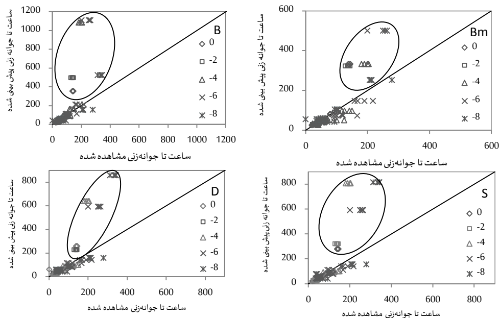
شکل ۳- زمان (ساعت) تا جواهر زنی پیش بینی شده با استفاده از توابع بتای اصلی (B)، بتای تغییر یافته (B m )، دندان مانند (D) و دو - تکه‌ای (S) در برابر مقادیر مشاهده شده در پتانسیل‌های مختلف آب (اعداد داخل شکل‌ها مربوط به پتانسیل آب بر حسب بار است و نقاط داخل بیضی مربوط به دمای ۵ درجه سانتی‌گراد است که در برازش خط مورد استفاده قرار نگرفتند).
