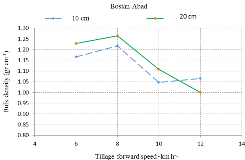
شکل ۴- جرم مخصوص ظاهری خاک در عمق‌های مختلف خاک‌ورزی- بستان‌آباد Fig. 4. Effect of tillage depth and forward speed on bulk density-Bostan-Abad
