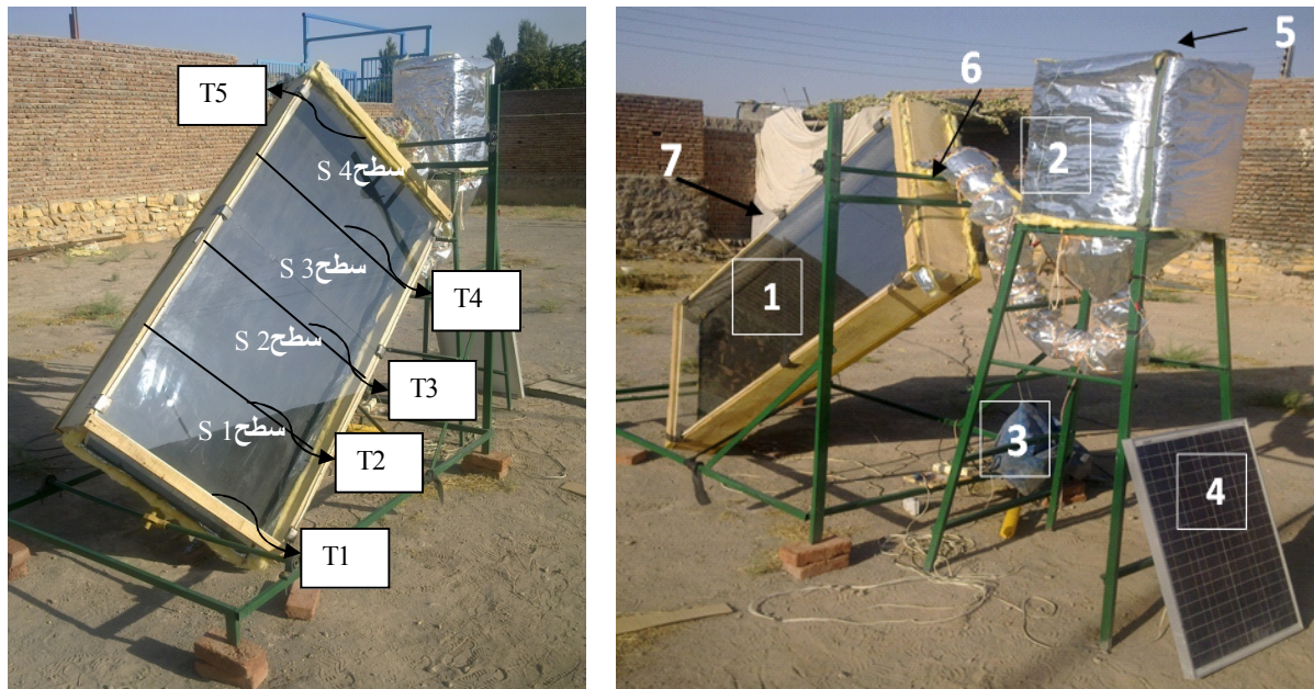
شکل ۲- خشک کن خورشیدی شامل صفحه جمع کننده، کابینت، پنل خورشیدی و سطوح مشخص شده برای آزمایش، (۱) صفحه جاذب، (۲) کابینت
