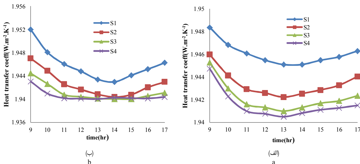
شکل ۵- تغییرات ضریب انتقال حرارت در سطوح مختلف از صفحه جمع کننده بر حسب زمان، (الف) با چرخش، (ب) بدون چرخش
