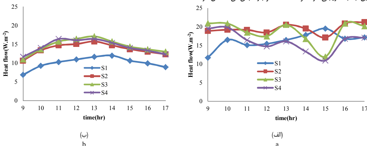
شکل ۶- تغییرات شار حرارتی در سطوح مختلف از صفحه جمع کننده بر حسب زمان، (الف) با چرخش، (ب) بدون چرخش
