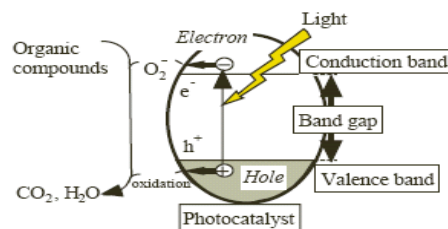
شکل ۱. مراحل انجام واکنش فتوکاتالیستی در سطح ذره کاتالیست
