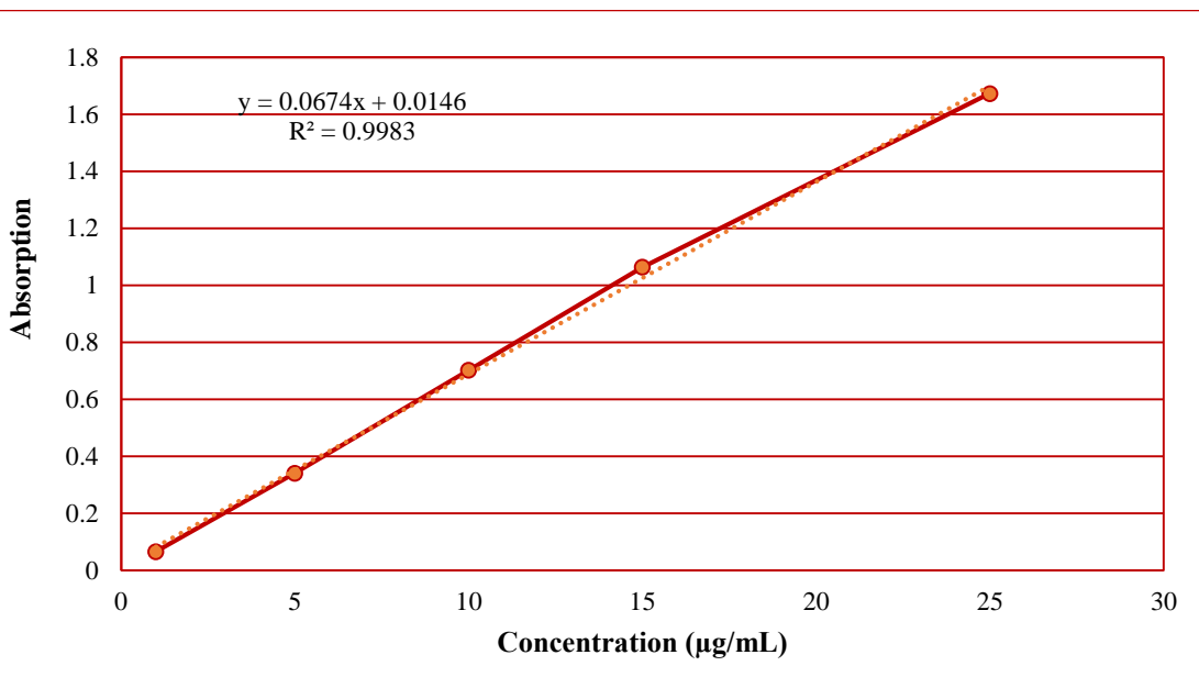
نمودار ۱- منحنی استاندارد نیستاتین در محلول آبی حاوی سدیم لوریل سولفات ۰/۲٪
