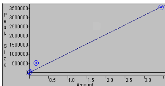
شکل (D-۱) - منحنی کالیبراسیون زایلن
