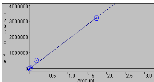
شکل (B-۱) - منحنی کالیبراسیون تولوئن
