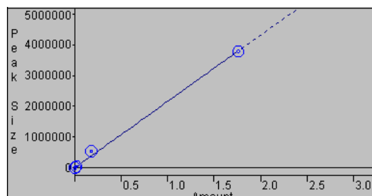
شکل (A-۱) - منحنی کالیبراسیون بنزن
