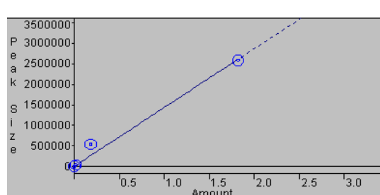
شکل (C-۱) - منحنی کالیبراسیون اتیل بنزن
