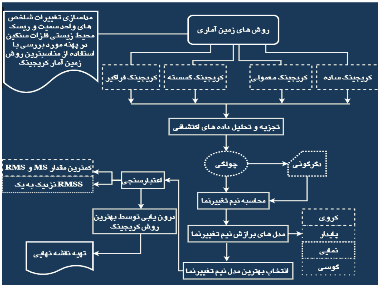
شکل ۱. ساختار مدل زمین آمار برای پیش بینی تغییرات شاخص های اکولوژیکی در منطقه مورد مطالعه
