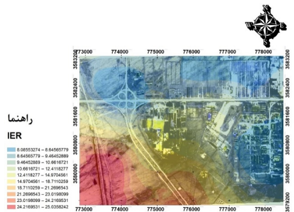
شکل ۴. نقشه توزیع مکانی شاخص ریسک محیط زیستی به روش
