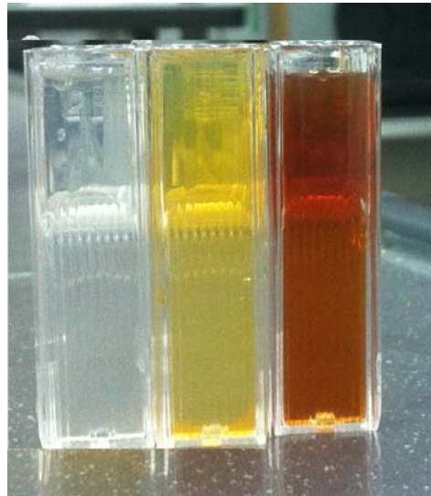
شکل ۱. سنتز نانوذرات نقره (نمونه سمت راست) که با تغییر رنگ عصاره پونه (نمونه وسط) بعد از اضافه کردن محلول نیترات نقره (نمونه سمت چپ) و قرار گرفتن در زیر نور آفتاب به مدت زمان ۳ دقیقه با چشم غیر مسلح قابل مشاهده است.
