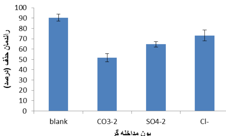
شکل ۸. راندمان حذف آلایندہ آنتیلین توسط نانولوله کربن مغناطیسی شده از محلول آبی با تاثیر یون های مختلف مداخله گر
