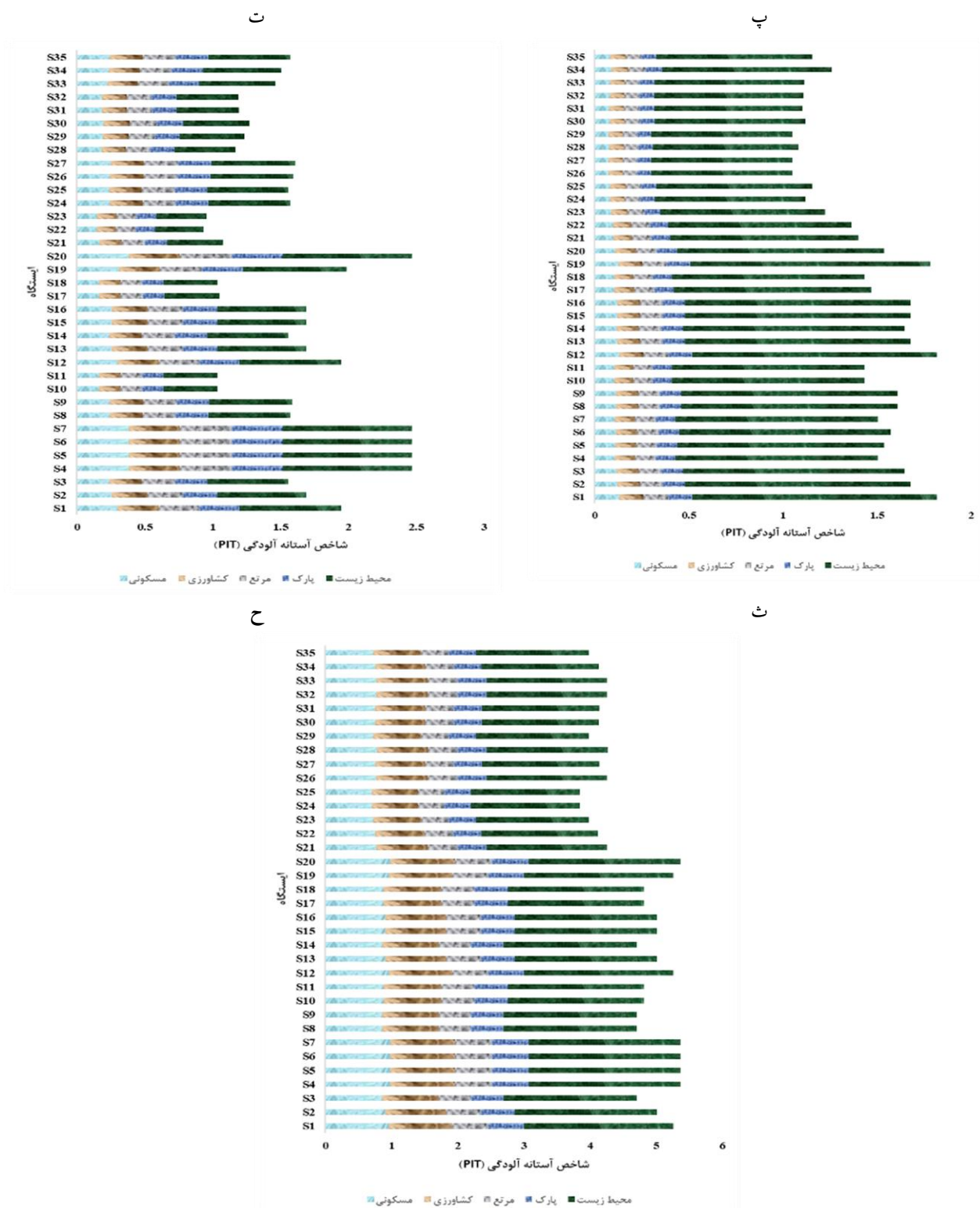
شکل ۴: نمودار تغییرات شاخص آستانه آلودگی (PIT) فلزات سنگین نیکل (الف)، مس (ب)، سرب (پ)، روی (ت)، مولیبدن (ث)، کبالت (ح) و آرسنیک
