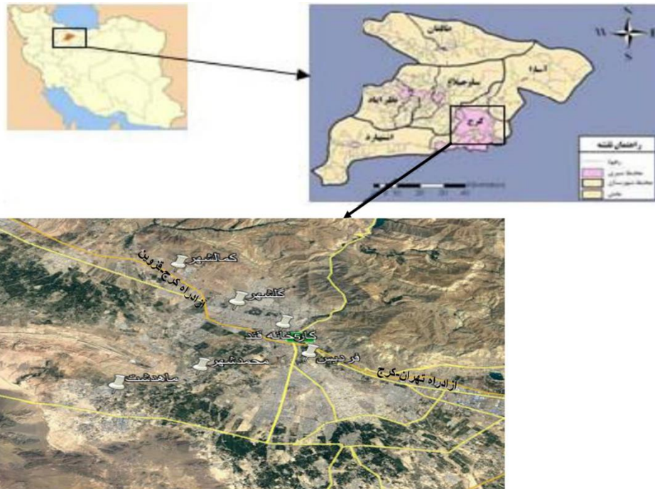
شکل ۱: موقعیت ایستگاه‌های نمونه‌برداری از نهشت اتمسفری شهر کرج
