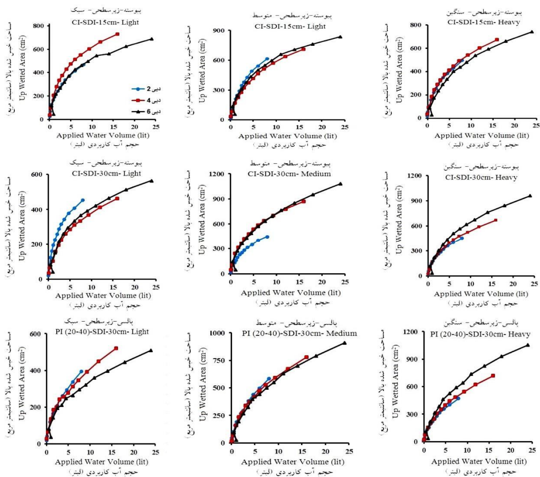
شکل ۷- تأثیر دبی قطره‌چکان بر روی مساحت خیس‌شدگی پیاز رطوبتی بالای قطره‌چکان در سیستم قطره‌ای با جریان پیوسته و پالسی.
