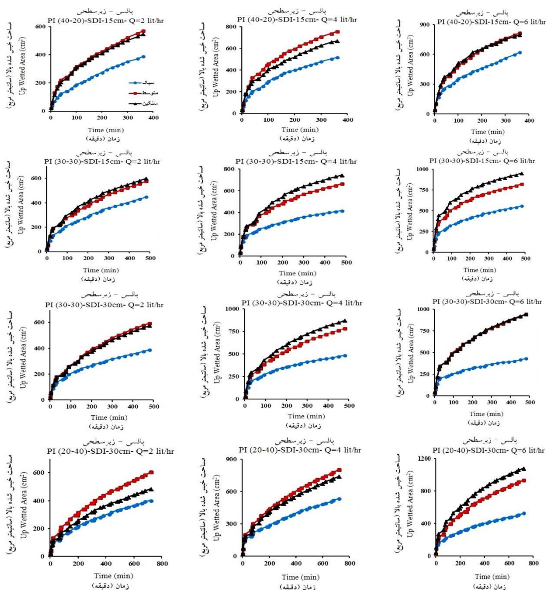
شکل ۹- تأثیر بافت خاک بر روی مساحت خیس‌شدگی پیاز رطوبتی بالای قطره‌چکان در سیستم قطره‌ای زیرسطحی با جریان پیوسته و پالسی.
