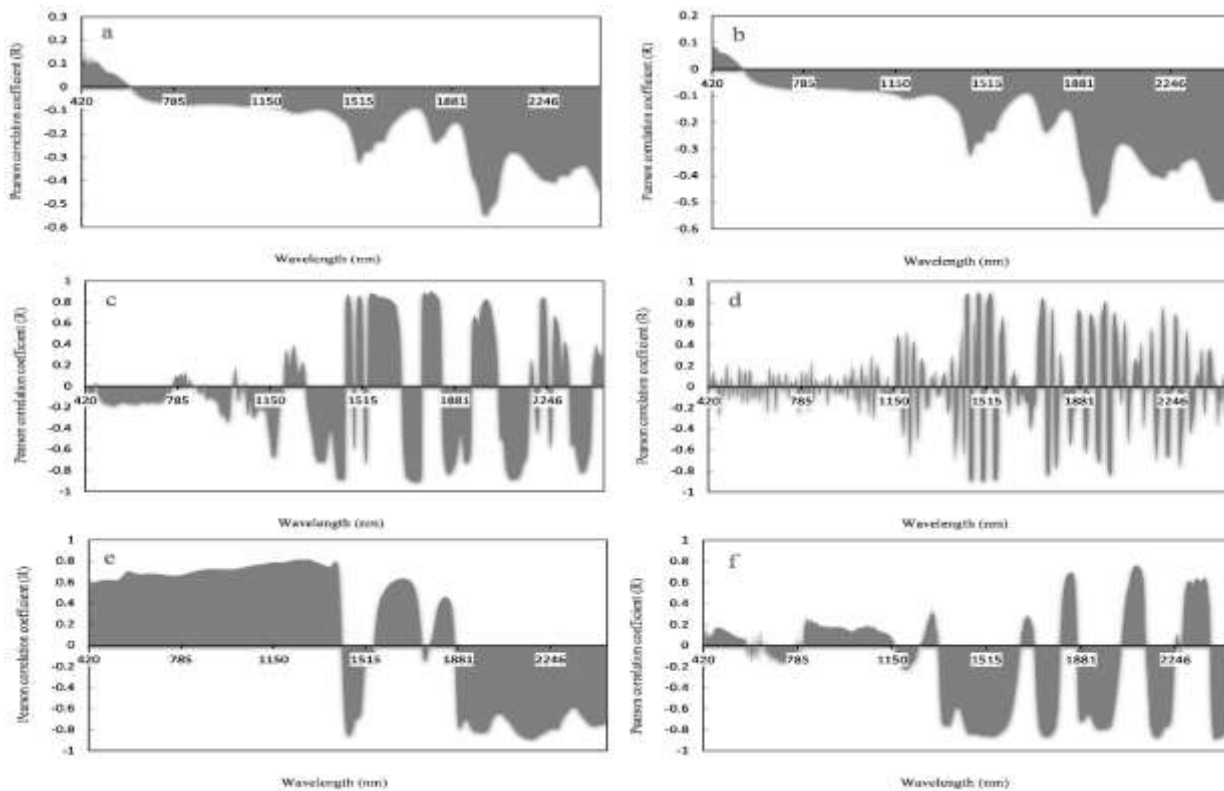
شکل ۳- نمودار همبستگی الگوی تغییرات بازتاب طیفی ناشی از تغییرات مقدار گچ خاک در طول موج‌های مختلف: a: طیف اصلی (ROW)، b: فیلتر ساویتزی گولای، c: مشتق اول همراه با فیلتر ساویتزی گولای (SD-SG)، d: مشتق دوم همراه با فیلتر ساویتزی گولای (FD-SG)، e: روش واریانس نرمال استاندارد (SNV)، f: حذف پیوستار (CR)
