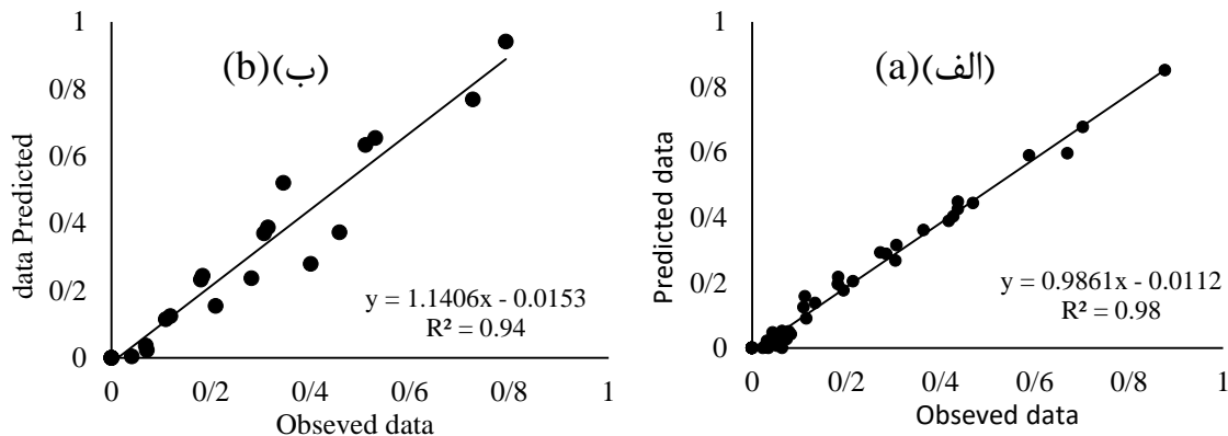
شکل ۳- مقایسه مقادیر مشاهده‌ای و برآوردشده شاخص MWD توسط مدل MLP برای داده‌های آموزشی (الف) و داده‌های آزمون (ب)
