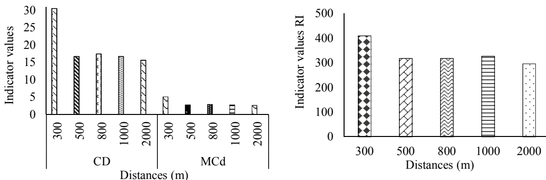
شکل ۴- وضعیت منطقه مورد مطالعه از نظر آلودگی فلزات سنگین با توجه به شاخص‌های CD، mCd و RI
