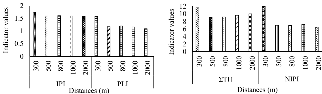
شکل ۳: وضعیت منطقه مورد مطالعه از نظر آلودگی فلزات سنگین با توجه به شاخص‌های IPI، PLI، PI_{Nemerow} و \Sigma TU Figure 3: Heavy metals pollution in the region according to PLI, IPI, PI_{Nemerow} and \Sigma TU indices
