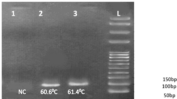
شکل ۴: الکتروفورز محصول PCR گرادیان دمایی Tm، برای ژن CXCL11 روی ژل آگارز ۱٪/۵. چاهک ۱: کنترل منفی (به جای cDNA از آب استفاده شد)، چاهک ۲ و ۳: محصول PCR بیمار سلولیک، L Ladder 50 bp (یکتا تجهیز آژما-شماره کاتالوگ YT8501). باند مورد نظر 109 bp می باشد.
