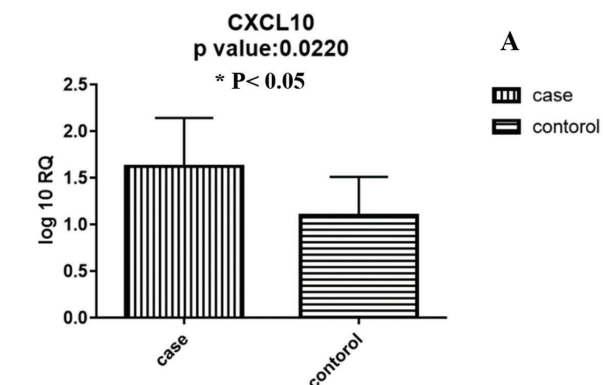
شکل ۸: میزان تغییرات بیان ژن‌های هدف در افراد مبتلا به سلولیک در مقایسه با افراد سالم. (A) تغییرات بیان ژن CXCL11 (B) تغییرات بیان ژن CXCL10.
