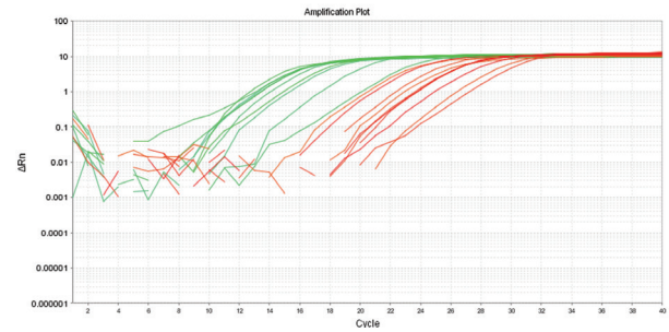
شکل ۶: منحنی تکثیر تصاعدی ژن‌های CXCL10 و B2M برحسب (سیکل-ΔRn) در بیماران مبتلا به سلولیک و افراد سالم.
