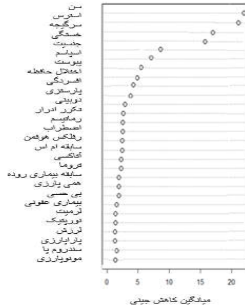
نمودار ۲: تعیین اهمیت متغیرها بر اساس میانگین کاهش جینی
