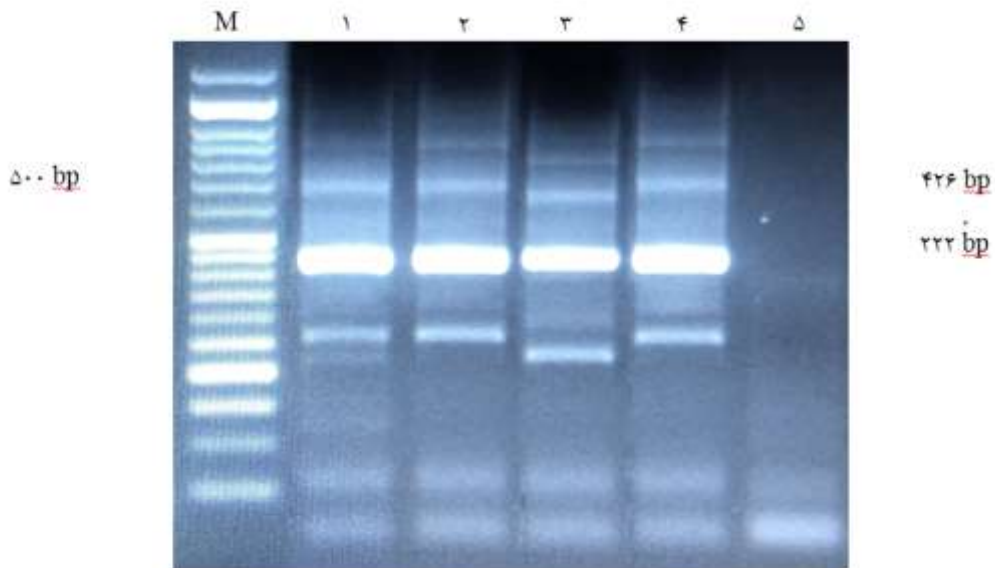
تصویر ۲- الکتروفورز محصولات Tetra-ARMA در بیماران سقط مکرر و گروه کنترل. در چاهک شماره ۱-۵ به ترتیب واجد ژنوتیپ‌های CT (۴۲۶ bp و ۲۲۲bp و ۲۵۹bp)، TT (۴۲۶ bp و ۲۵۹bp)، CC (۴۲۶ bp و ۲۲۲bp)، TT (۴۲۶ bp و ۲۵۹bp) و ۵۰۰ bp (۲۵۹bp و ۴۲۶ bp) و کنترل منفی (NTC)، در افراد بیمار مشاهده شد.
