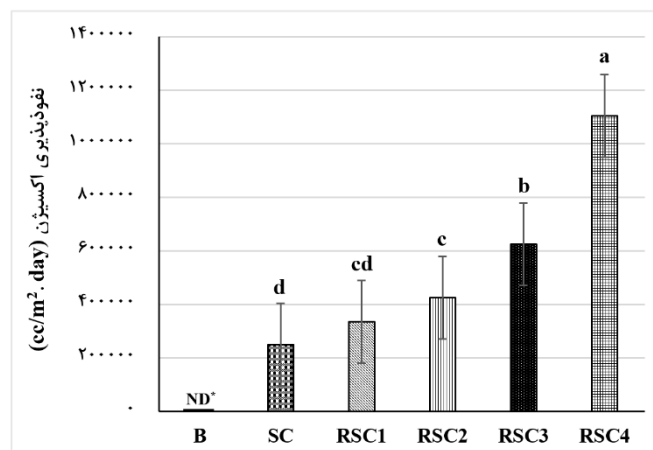
شکل ۲- میزان نفوذپذیری اکسیژن در مقوای بدون پوشش و پوشش‌دار (ND* اندازه‌گیری انجام نشده است)
