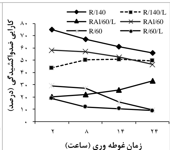
شکل ۶- اثر اصلاح بر کارایی ضدواکنش‌دهی طی آزمون غوطه‌وری در آب
