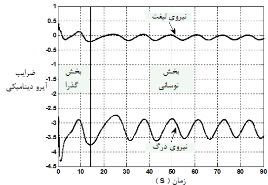
شکل ۱۱- ضرایب لیفت و پسا نسبت به زمان برای کلکتور تنها (کلکتور نسبت به باد دارای زاویه صفر می باشد)
