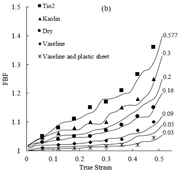
شکل ۱۲- نمودار کالیبراسیون استوانه بلند سربی به همراه داده‌های تجربی روان کارهای مختلف، الف) ضریب بشکه‌ای شدن هندسی، ب) ضریب بشکه‌ای شدن نیرویی.
