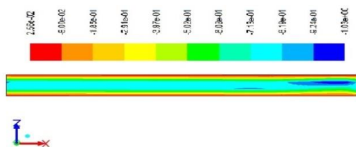
شکل ۶- سرعت V_x در مرکز کانال در جهت X
