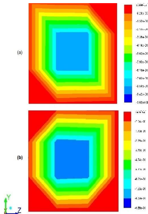
شکل ۴- سرعت V_x در مرکز کانال در صفحه Y-Z در دو حالت (a) و (b) n=2400rpm و n=1800rpm
