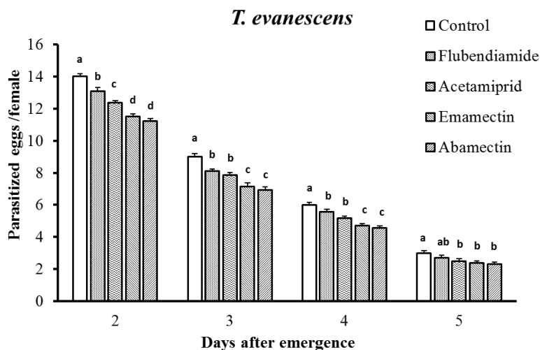
شکل ۲. میانگین شمار تخم‌های پارازیت‌دهنده به وسیله زنبور Trichogramma evanescens در روزهای گوناگون پس از پیدایش زنبور در تیمار با LC_{25} آفت‌کش‌های گوناگون. حرف‌های متفاوت نشان‌دهنده وجود اختلاف معنی‌دار در P<0/01 هستند.
