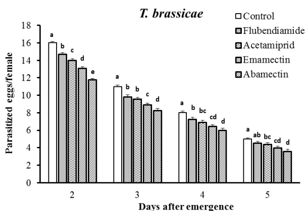
شکل ۱. میانگین شمار تخم‌های پارازیت‌شده به‌وسیله زنبور Trichogramma brassicae در روزهای گوناگون پس از پیدایش زنبور در تیمار با LC 25 آفت‌کش‌های گوناگون. حرف‌های متفاوت نشان‌دهنده وجود اختلاف معنی‌دار در P < 0.05 هستند.
