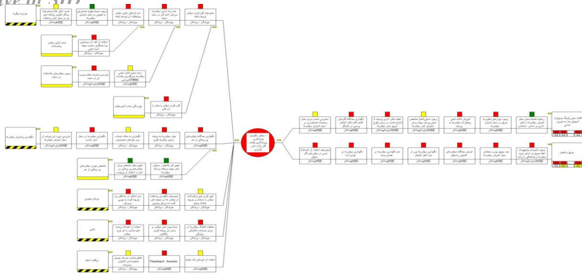
نمودار ۲: نمودار پاپیونی پیامد سیلندرهای تحت فشار، جوشکاری و برشکاری با گاز
