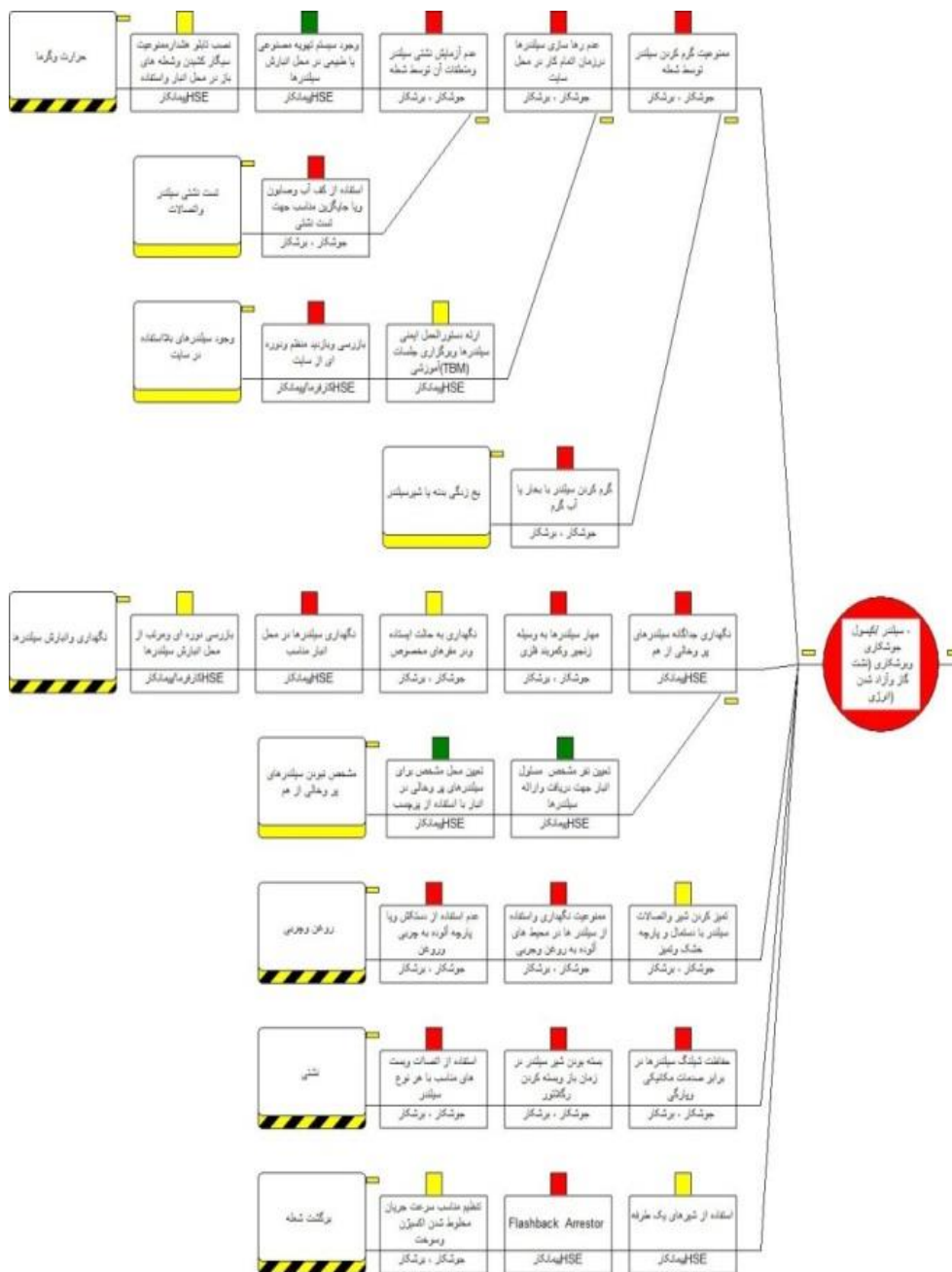
نمودار ۱: نمودار پاپیونی تهدید سیلندرهاي تحت فشار، جوشکاری و برشکاری با گاز
