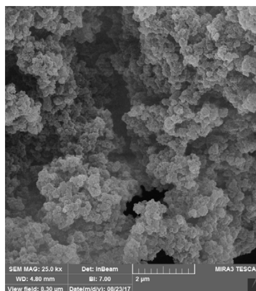
شکل (۱) - تصویر میکروسکوپی (SEM) مربوط به ساختار و اندازه سطوح پلیمر قالب مولکولی سنتز شده برای پرمترین
