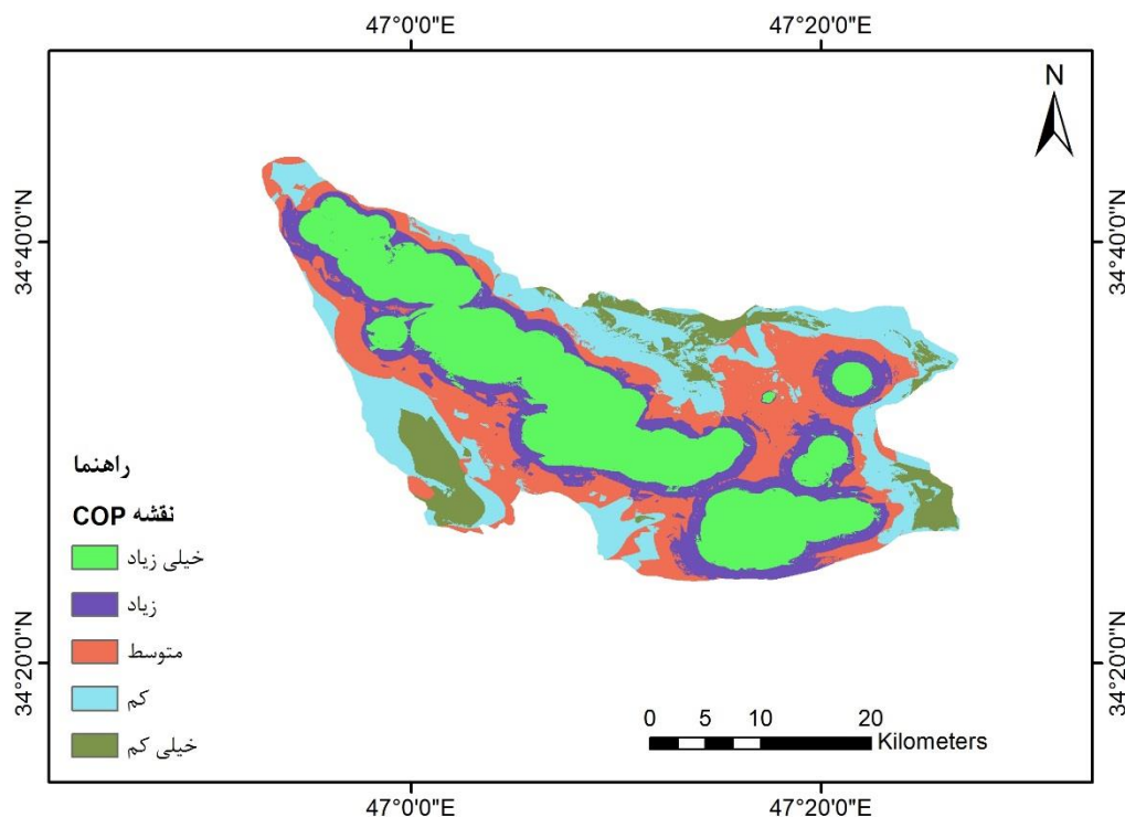
شکل ۱۰. نقشه آسیب پذیری آبخوان آژوان-بیستون بر اساس روش COP
