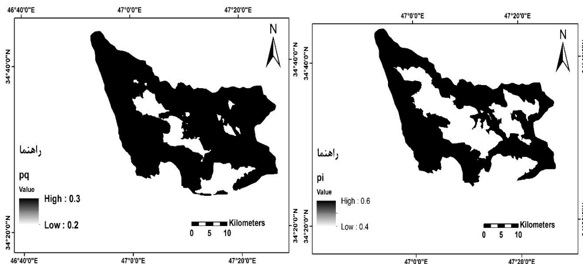
شکل ۸. نقشه مقدار بارش (Pi) و توزیع زمانی بارش (Pq) منطقه مورد مطالعه
