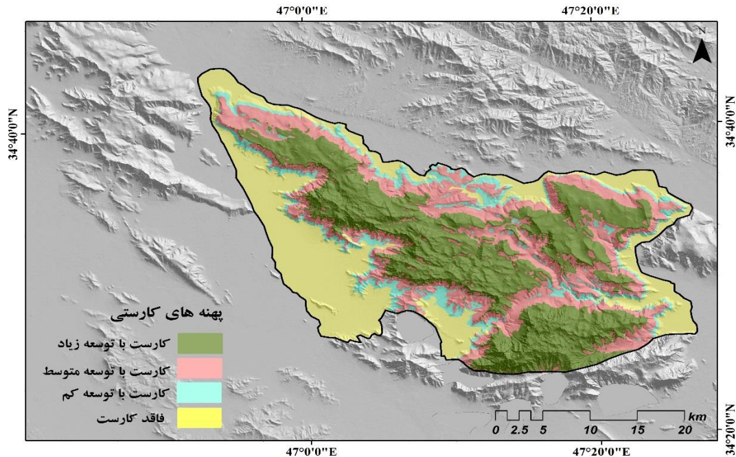
شکل ۳. نقشه پهنه‌بندی توسعه کارست سطحی مدل فازی توده بیستون
