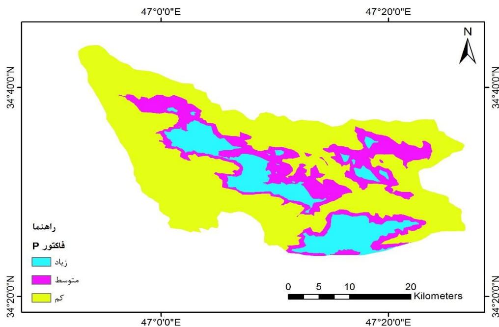
شکل ۹. نقشه پهنه‌بندی فاکتور P
