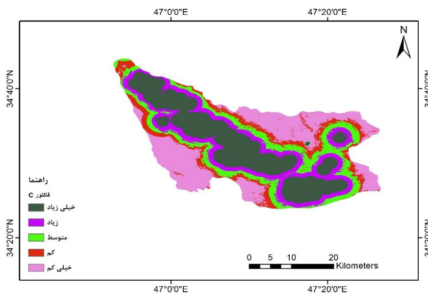
شکل ۵. نقشه پهنه‌بندی فاکتور C
