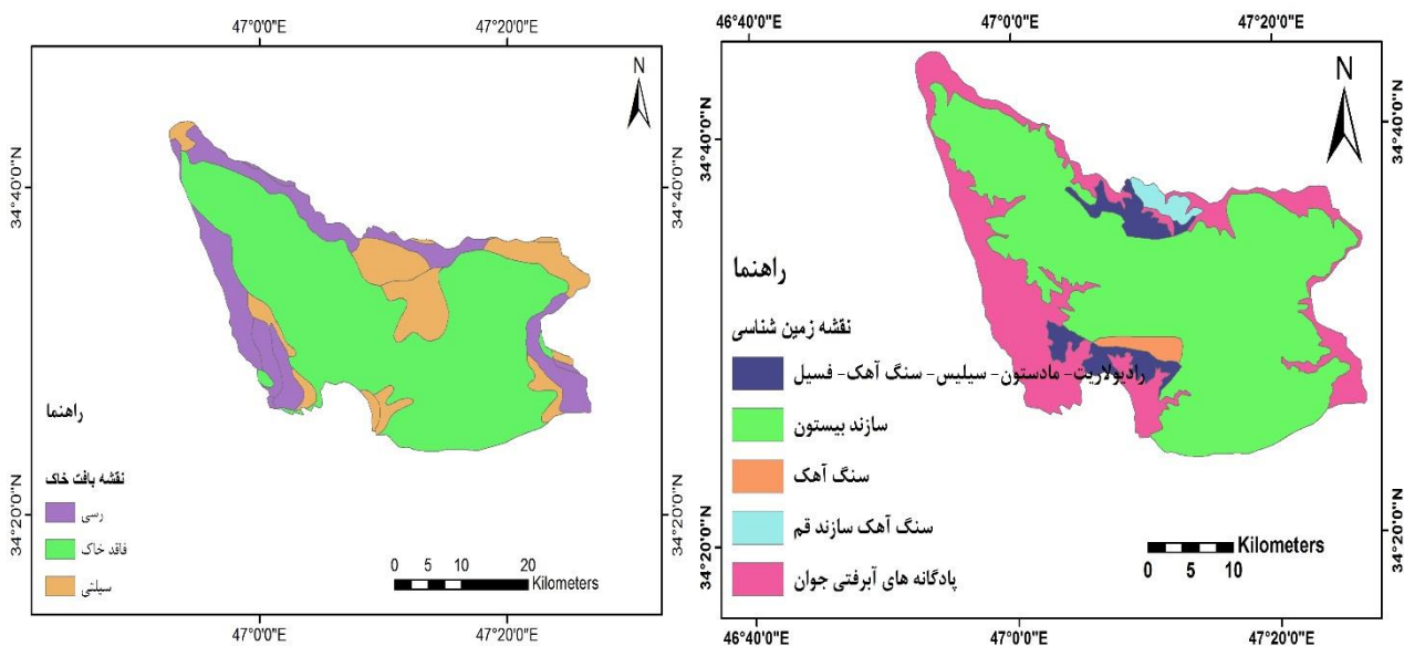
شکل ۶. نقشه بافت خاک و زمین‌شناسی منطقه مورد مطالعه
