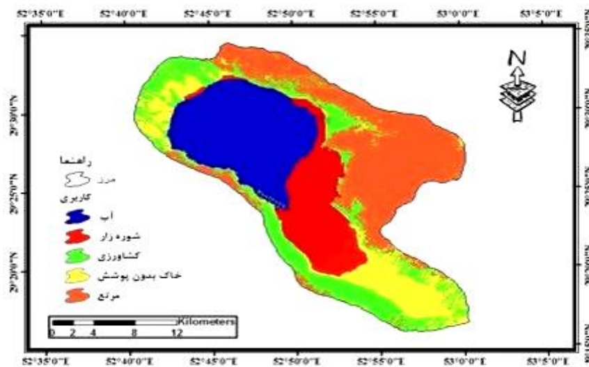
شکل ۴. نقشه کاربری اراضی با استفاده از الگوریتم حداکثر شباهت (MLC) سال ۱۳۸۱
