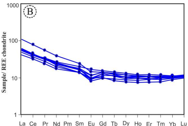
شکل ۹- A) عنصرهای فرعی در سنگ‌های نفوذی منطقه در نمودار عنکبوتی بهنجارشده در برابر ترکیب گوشته اولیه (Sun and McDonough, 1989)؛ B) عنصرهای خاکی کمیاب سنگ‌های نفوذی منطقه رنجرز در نمودار بهنجارشده به ترکیب کندریت (Boynnton, 1984)
