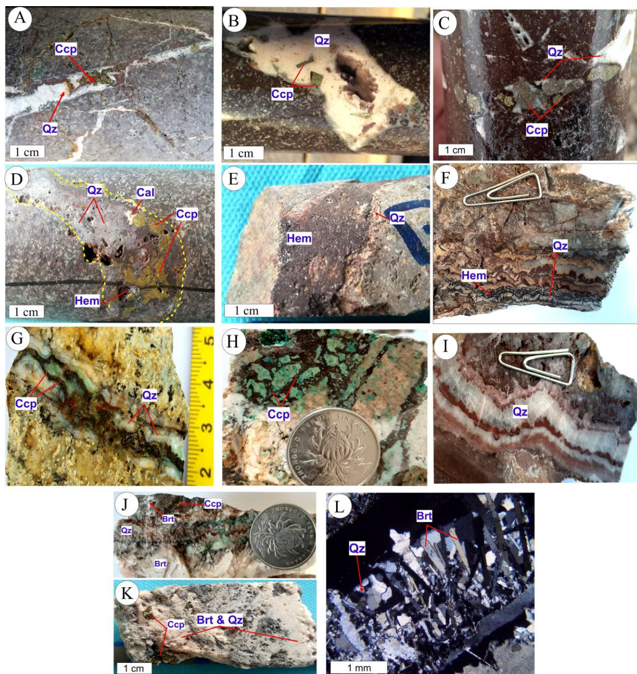
شکل ۱۲- (A) نمایی از یک رگچه کوارتز- کالکوپیریت؛ (B) کانی‌سازی رگه‌ای کوارتز- کالکوپیریت؛ (C) نمایی از یک رگه کوارتز- کالکوپیریت که دچار زمین‌ساخت کششی شده است؛ (D) رگه کوارتز- کلسیت- کالکوپیریت- اسپیکولارهماتیت؛ (E) رگه کوارتز- اسپیکولارهماتیت؛ (F) کانی‌سازی اسپیکولارهماتیت- کوارتز به‌صورت قشری- کلوform؛ (G) نمایی از کانی‌سازی کالکوپیریت- کوارتز به صورت قشری- کلوform؛ (H) نمایی از یک برش گرمایی با قطعات توف آندزیتی و سیمانی از بقایای کالکوپیریت در زمینه‌ای از اکسیدهای ثانویه مس؛ (I) نمایی از حضور کوارتز با بافت قشری در منطقه؛ (J, K) نمایی از هم‌رشدی باریت- کوارتز همراه با کالکوپیریت؛ (L) نمایی از هم‌رشدی باریت- کوارتز در مقطع میکروسکوپی (نام اختصاری کانی‌ها (Whitney and Evans, 2010): Ccp: کالکوپیریت؛ Qz: کوارتز؛ Hem: هماتیت؛ Cal: کلسیت؛ Brt: باریت)
