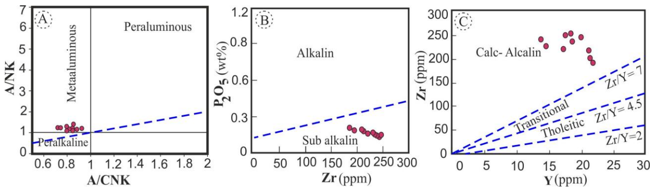
شکل ۷- A) نمودار تعیین شاخص آلومینیم (Shand, 1943)؛ B) شناسایی سری ماگمایی در نمودار P_2O_5 در برابر Zr در برابر Zr (Winchester and Floyd, 1977)؛ C) تفکیک سری‌های ماگمایی سنگ‌های منطقه در نمودار Zr در برابر Y (Ross and Bedard, 2009)
