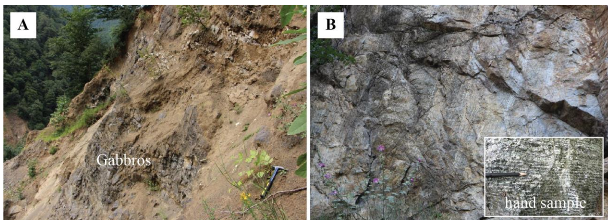
شکل ۲- (A) نمای از رخنمون گابروها در روستای گیلونده‌رود؛ (B) نمای از رخنمون گابروها با لایه‌بندی آذرین در روستای زودل
