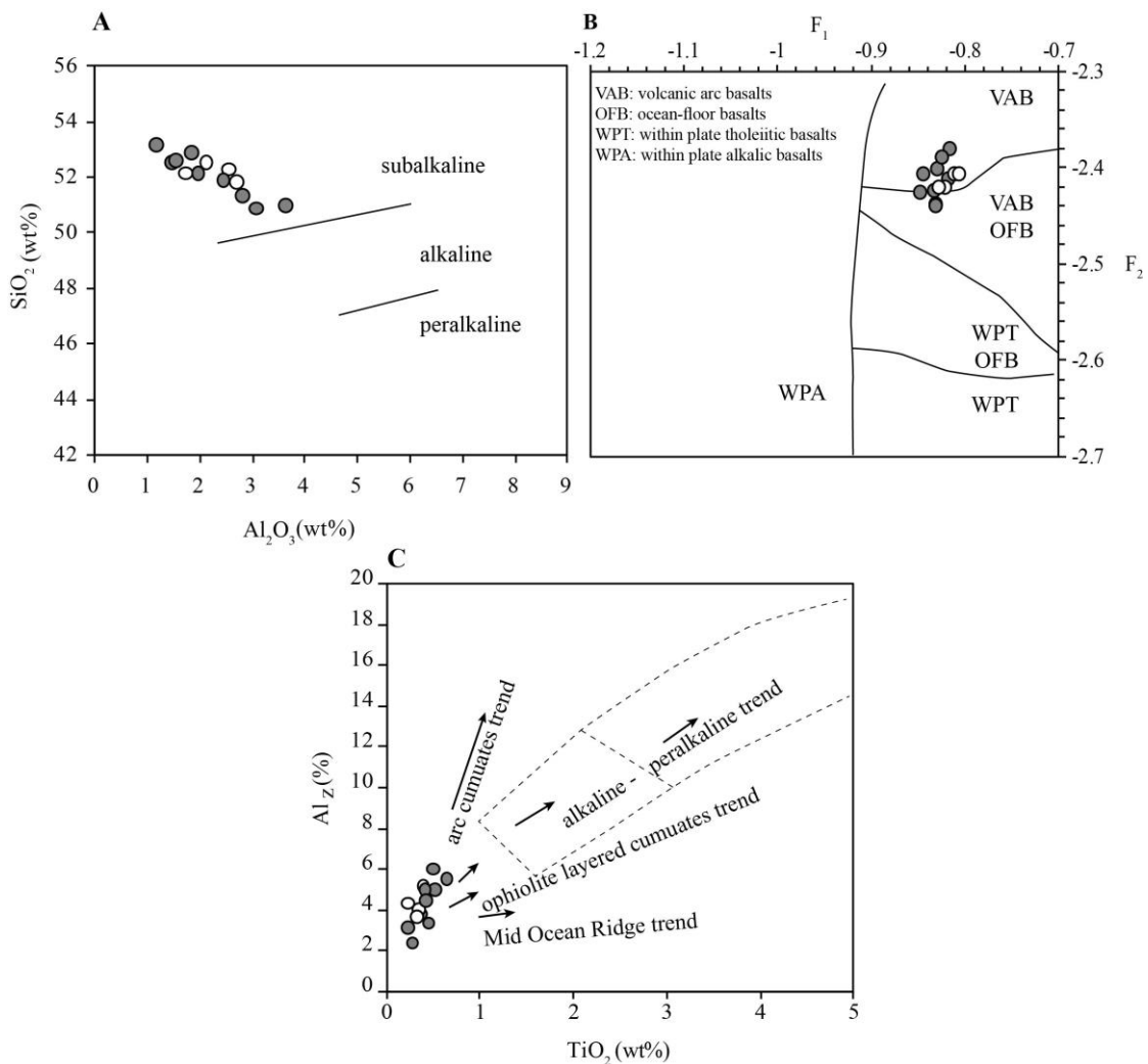
شکل ۵- شناسایی سری ماگمایی مذاب مادر و پهنه زمین‌ساختی پیدایش گابروهای گشت-ماسوله برپایه شیمی کلینوپیروکسن در: (A) نمودار Al_2O_3 در برابر SiO_2 برپایه ترکیب شیمیایی کانی کلینوپیروکسن (Le Bas, 1962)؛ (B) نمودار F_1 در برابر F_2 (Nisbet and Pearce, 1977)؛ (C) نمودار TiO_2 در برابر Al_z (Loucks, 1990) (نماد کانی‌ها همانند شکل ۴ است)
