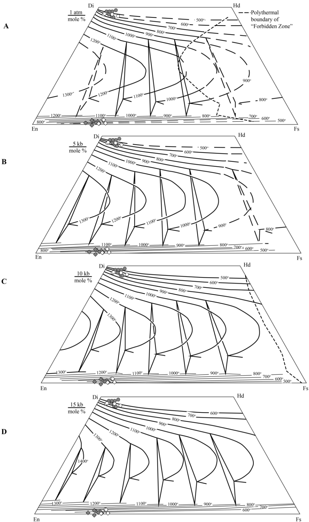
شکل ۷- A تا D) سنجش کمترین دمای تبلور کانی ارتوپیروکسن و کلینوپیروکسن در گابروهای منطقه گشت-ماسوله بر پایه دماسنج گرافیکی پیشنهادی Lindsley (۱۹۸۳) در فشارهای یک اتمسفر تا ۱۵ کیلوپار (نماد کانی‌ها همانند شکل ۴ است)
