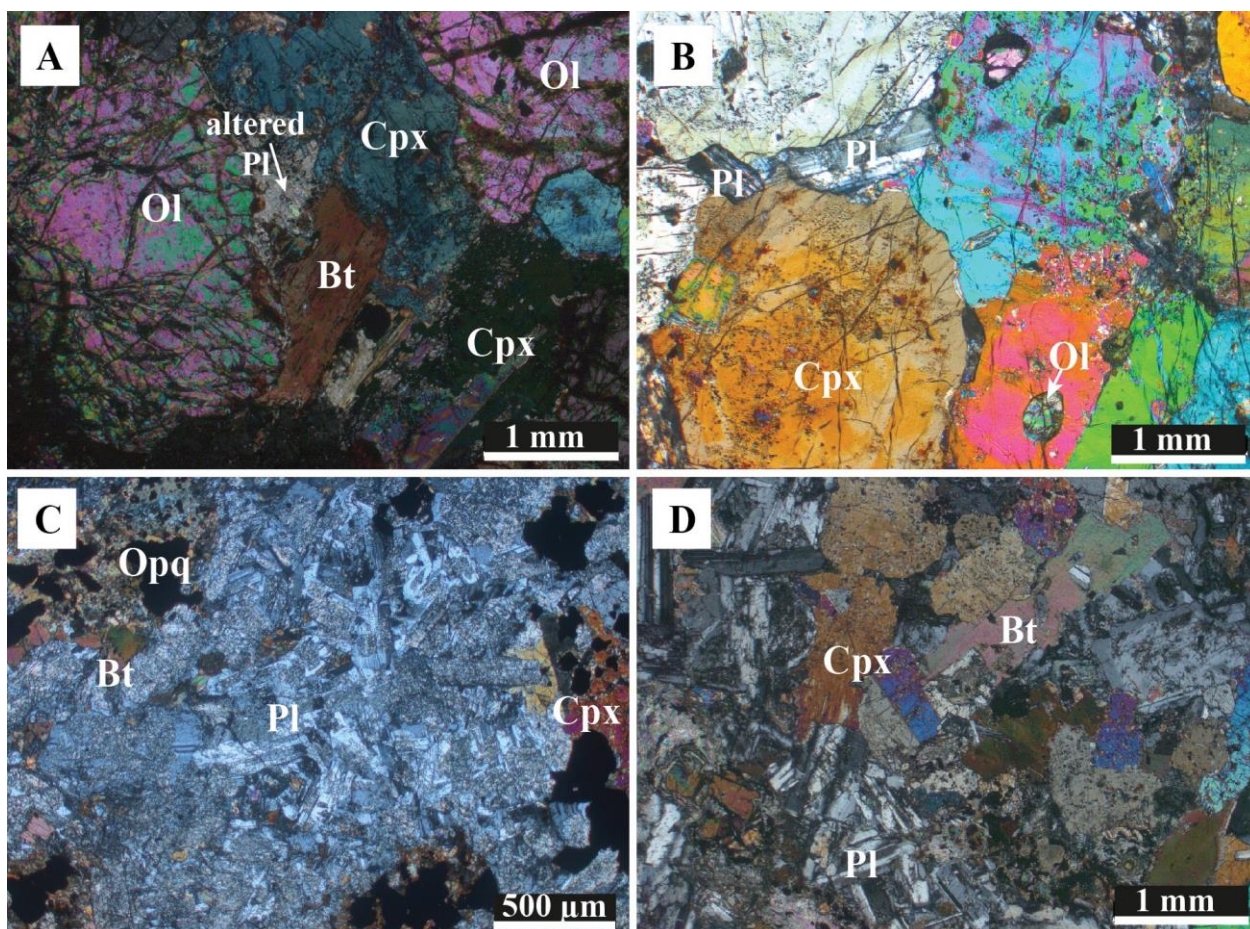
شکل ۳- تصویرهای میکروسکوپی از: A، B) گابروی کومولایی منطقه گشت-ماسوله. پلاژیوکلاز کانی اینترکومولوس است و فضای میان دانه‌های درشت الیوین و کلینوپیروکسن را پر کرده است. در تصویر B، الیوین به صورت میانبار در کلینوپیروکسن دیده می‌شود؛ C) پلاژیوکلاز فراوان‌ترین کانی در لایه‌های روشن است و کلینوپیروکسن، بیوتیت و اکسیدهای آهن و تیتانیم در لایه‌های تیره انباشته شده‌اند (گابروی سرشار از پلاژیوکلاز در روستای زودل؛ این تصویری از مقطع نازک نمونه دستی در شکل ۲- A است)؛ D) گابروی ایزوتروپ منطقه گشت-ماسوله (نام اختصاری کانی‌ها برگرفته از Whitney و Evans (۲۰۱۰) است)
