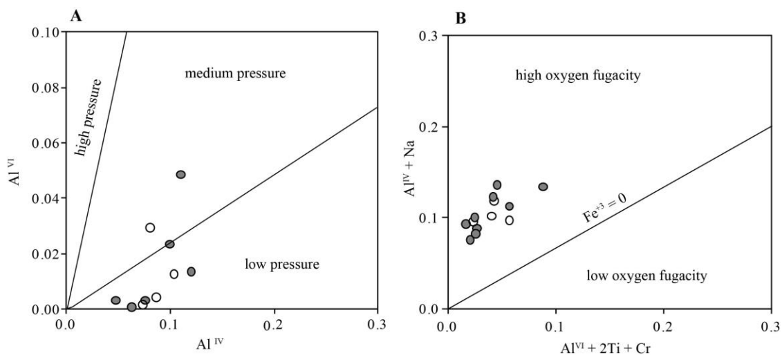
شکل ۶- A) نمودار Al^{IV} در برابر Al^{VI} برای ارزیابی محدوده فشار تبلور کانی کلینوپیروکسن از ماگمای مادر سنگ‌های گابرویی منطقه گشت-ماسوله (Aoki and Shiba, 1973)؛ B) نمودار Al^{IV}+Na در برابر Al^{VI}+2Ti+Cr برای ارزیابی شرایط اکسیداسیون تبلور کانی کلینوپیروکسن از ماگمای مادر گابروهای بررسی شده (Schweitzer et al. , 1974) (نماد کانی‌ها همانند شکل ۴ است)
