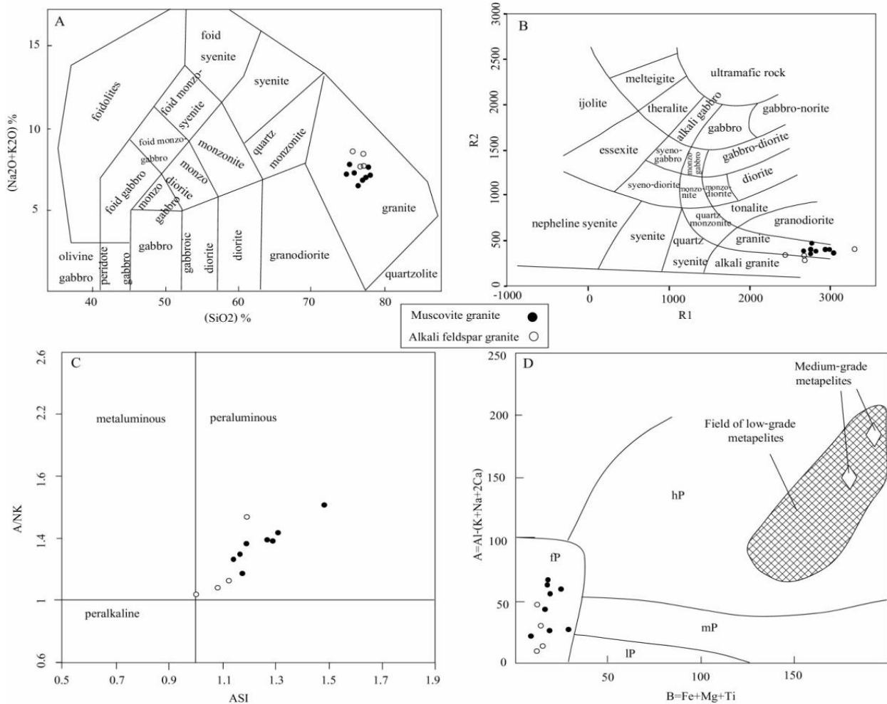
شکل ۴- ترکیب مسکوویت گرانیت‌ها و آلکالی‌فلدسپارگرانیت‌های گرمی‌چای در: (A) نمودار SiO 2 در برابر Na 2 O+K 2 O برای رده‌بندی سنگ‌های آذرین درونی (Middlemost, 1994)؛ (B) R1 در برابر R2 برای رده‌بندی سنگ‌های آذرین درونی (De Shand, 1979)؛ (C) نمودار A/NK در برابر ASI (La Roche et al., 1979)؛ (D) رده‌بندی شیمیایی سنگ‌های پرآلومینوس (Villaseca et al., 1998)؛ (hP: highly peraluminous; mP: moderately peraluminous; IP: low peraluminous; fP: highly felsic peraluminous)
