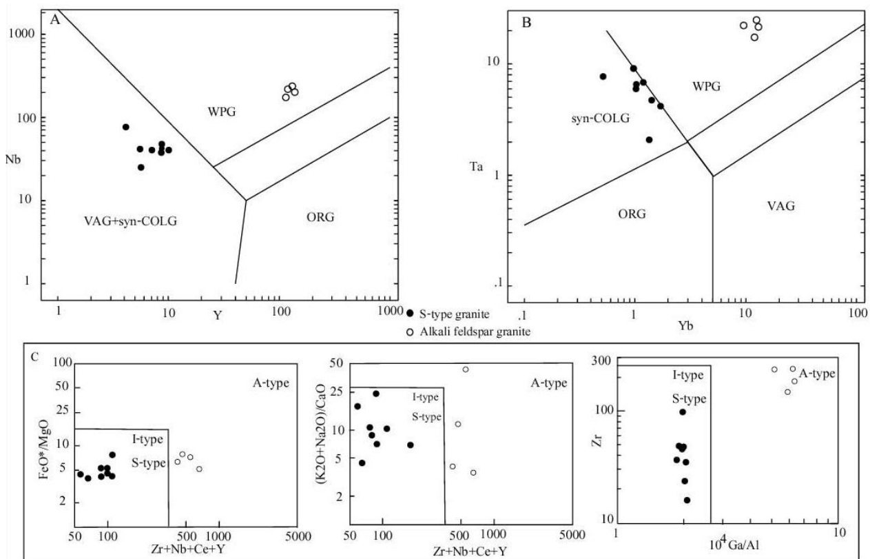
شکل ۷- مسکوویت گرانیت ها و آلکالی فلدسپار گرانیت های گرمی چای در: A, B) نمودارهای شناسایی پهنه زمین ساختی (Pearce et al., 1984); C) نمودارهای پیشنهادی Whalen و همکاران (۱۹۸۷) برای شناسایی گرانیت های S-type, I-type و type
