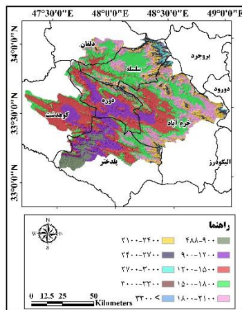
طبقات ارتفاع
