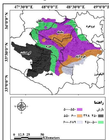
بارش
