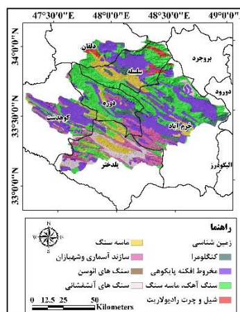
زمین شناسی
