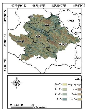
شیب
