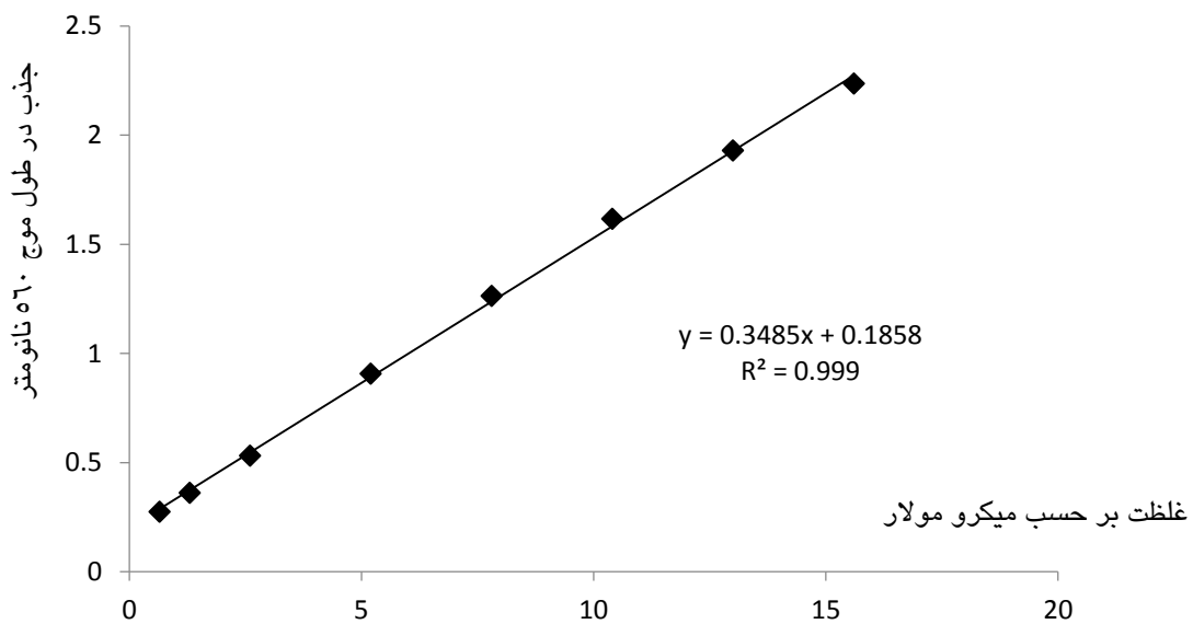
شکل ۱ - نمودار منحنی کالیبراسیون با غلظت‌های ۱۵/۶-۰/۶۵ میکرومولار از سدیم دی تیونیت استاندارد
