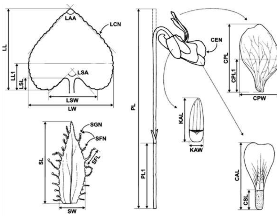
شکل ۱. ویژگی های مورفولوژی اندازه گیری شده برگرفته شده از مقاله (2008) Hodalova et al.
