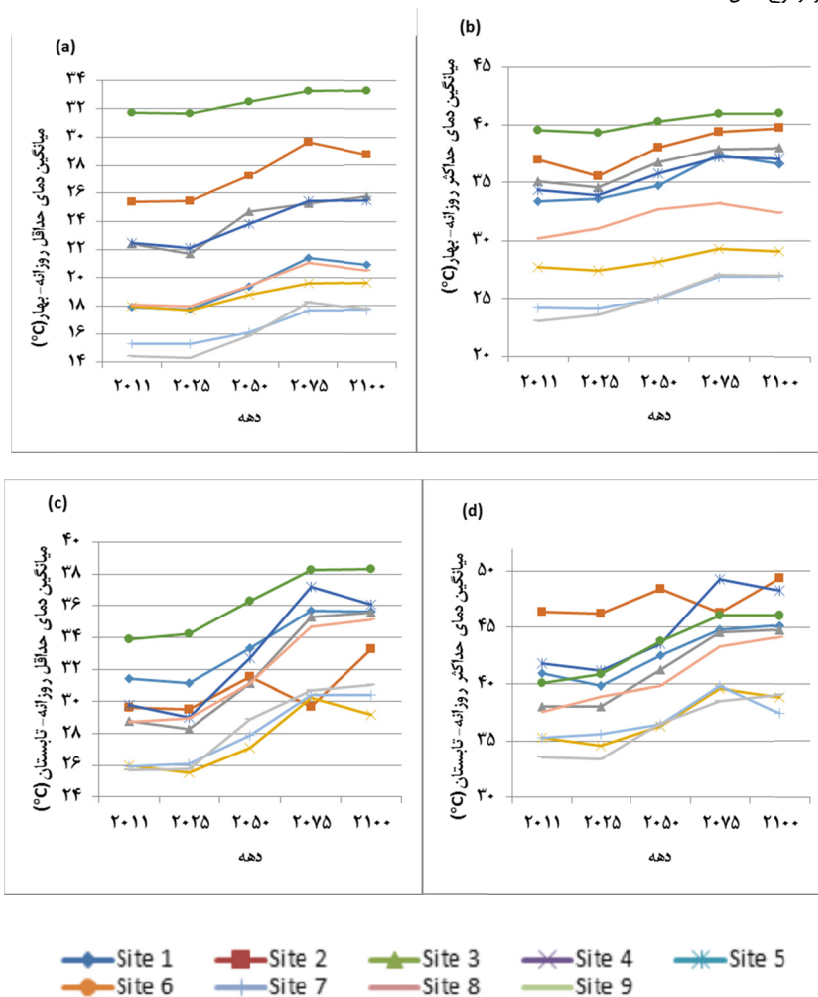
شکل ۲- تغییرات میانگین دمایی حداقل و حداکثر روزانه در فصل بهار و تابستان در دهه های آتی بر اساس پیش بینی مدل " (a) روند تغییرات دمایی حداقل روزانه در فصل بهار؛ (b) روند تغییرات دمایی حداکثر روزانه در فصل بهار؛ (c) روند تغییرات دمایی حداقل روزانه در فصل تابستان؛ (d) روند تغییرات دمایی حداکثر روزانه در فصل تابستان)
